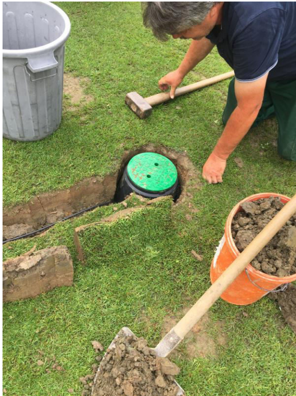
Nivellierung der Beregnungsbox
